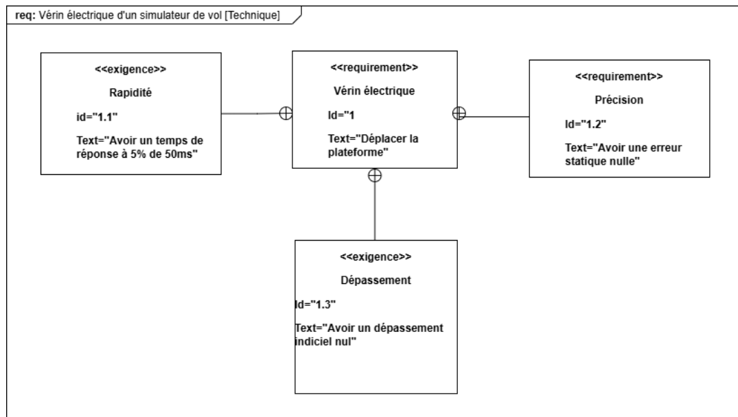
Figure 3: Extrait du diagramme des exigences du vérin électrique
